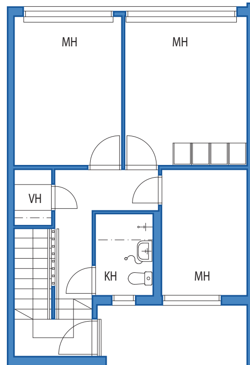
2. KERROS
