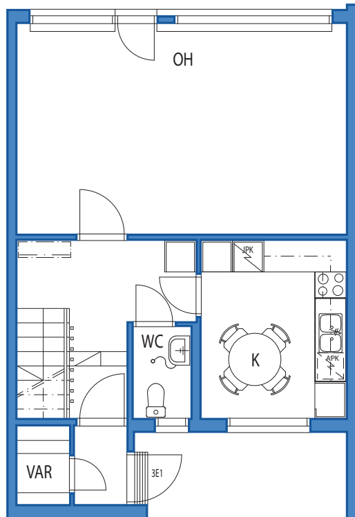
1. KERROS
