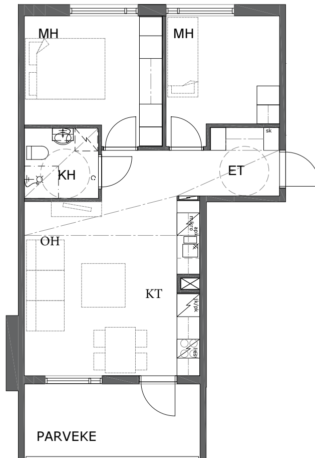
POHJAPIIRROS 1/100
