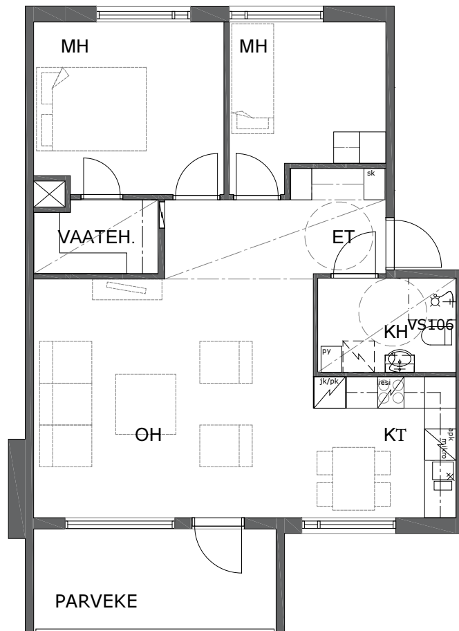
POHJAPIIRROS 1/100
