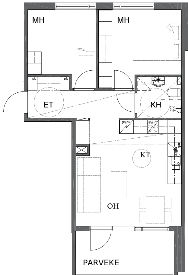
POHJAPIIRROS 1/100
