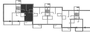
SIJAINTIPIIRROS (1.KERROS)
