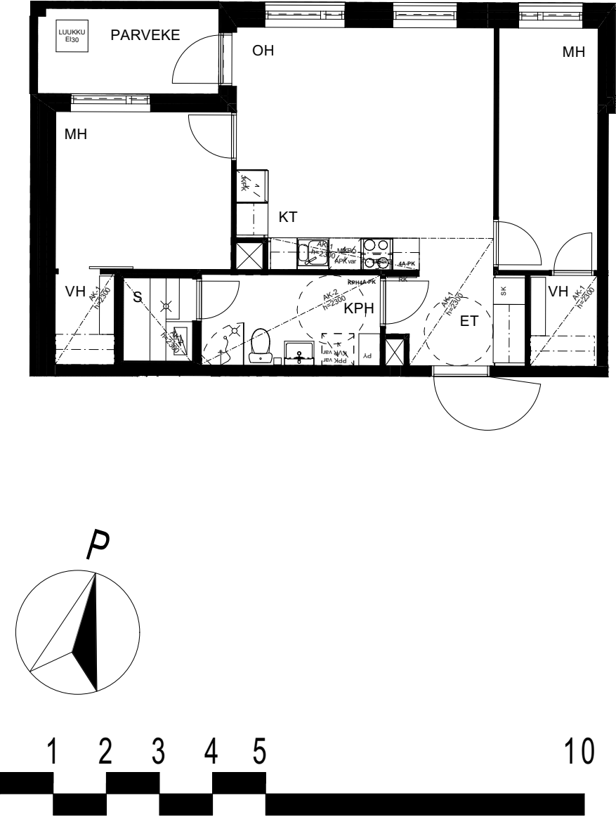
Mittakaava 1:100
